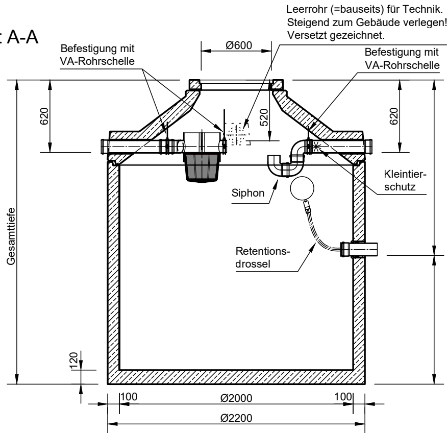
Grundriss
